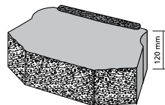
Ansicht Trockenmauerstein Unterseite mit Versatzlippe
