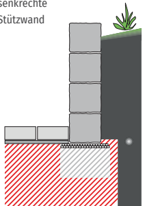
geneigte Stützwand
