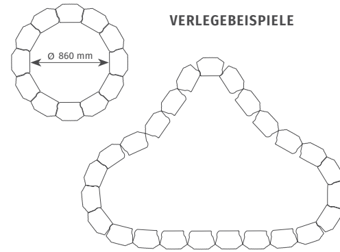
VILA FLOR TROCKENMAUERSTEIN grau
